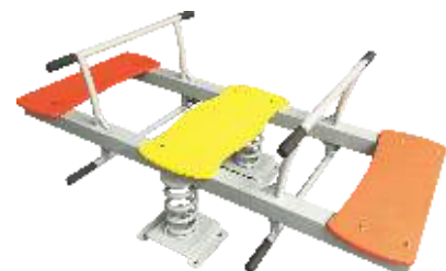
ZM-D115 多人跷跷板 规格size: 250×39×107cm 价格price: 15000元
