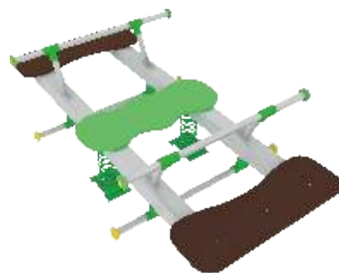
ZM-D114 多人跷跷板 规格size: 250×39×107cm 价格price: 15000元
