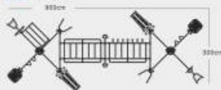
12柱双梯字形
